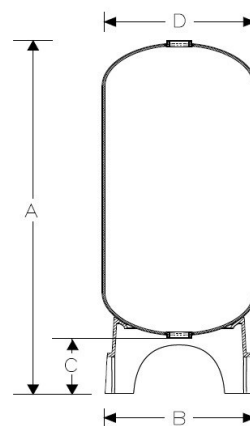
三角底座
