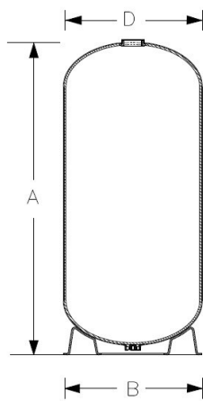
標準底座
